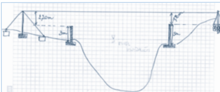
Schets van de nieuw te bouwen oversteek over de Rio Verde
